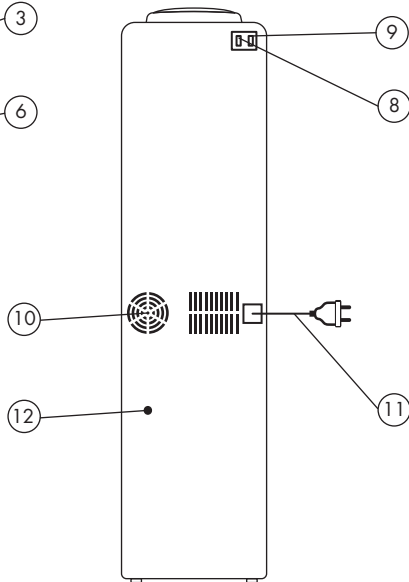
Артқы көрініс
