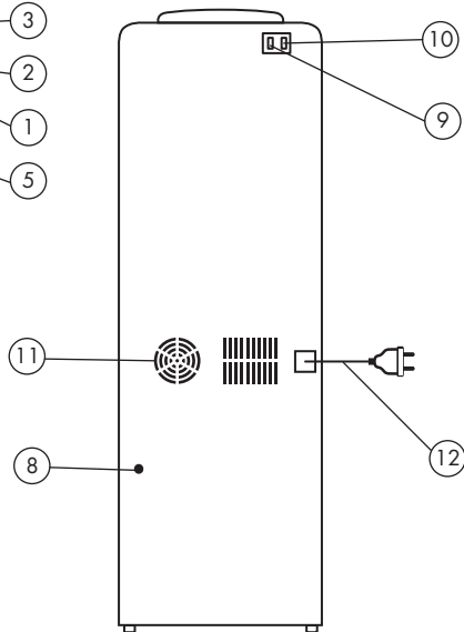
Вид сзади
